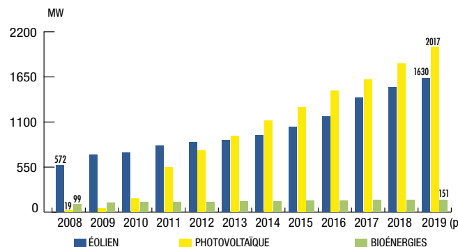
Evolution capacités installées 2008-2019
