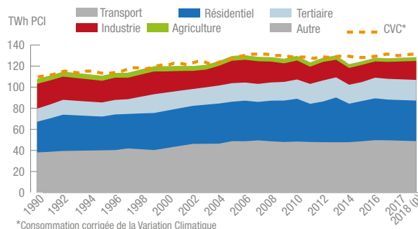
Évolution de la consommation d'énergie finale par secteur
