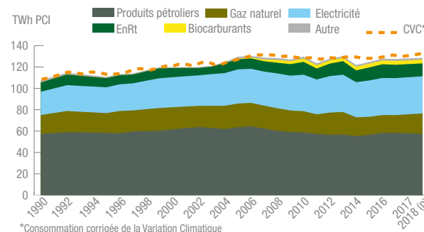
Évolution de la consommation d'énergie finale par énergie
